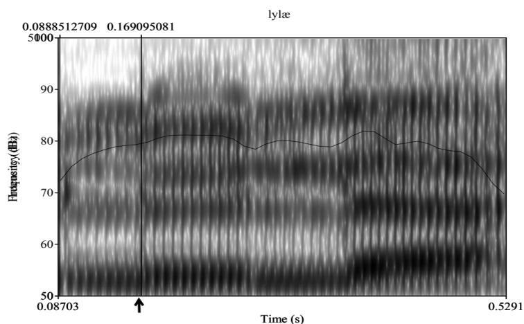
شکل (۱) طیف‌نگاشت زنجیره آوایی /ly.læ/ تولیدشده توسط یکی از گویشوران مرد است. پایان [I] در این طیف‌نگاشت توسط پیکان مشخص شده است.
