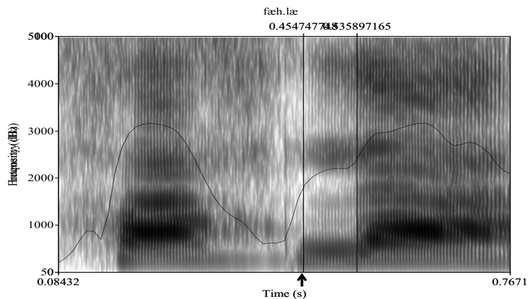
شکل (۵) طیف‌نگاشت مربوط به زنجیره آوایی /fæh.læ/ تولیدشده توسط یکی از گویشوران زن است. آغاز [1] در این طیف‌نگاشت توسط پیکان مشخص شده است.
