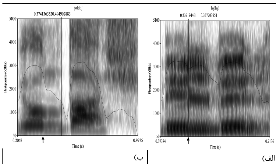
شکل (۷) طیف‌نگاشت (الف) مربوط به زنجیره آوایی /byl.byl/ تولیدشده توسط یکی از گویشوران مرد است.
