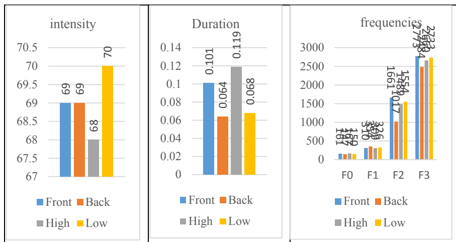
شکل (۶) میانگین فرکانس سازه‌های اول، دوم و سوم [1] بر اساس واکه پس از آن در جایگاه آغاز هجا بعد از همخوان بی‌واک
