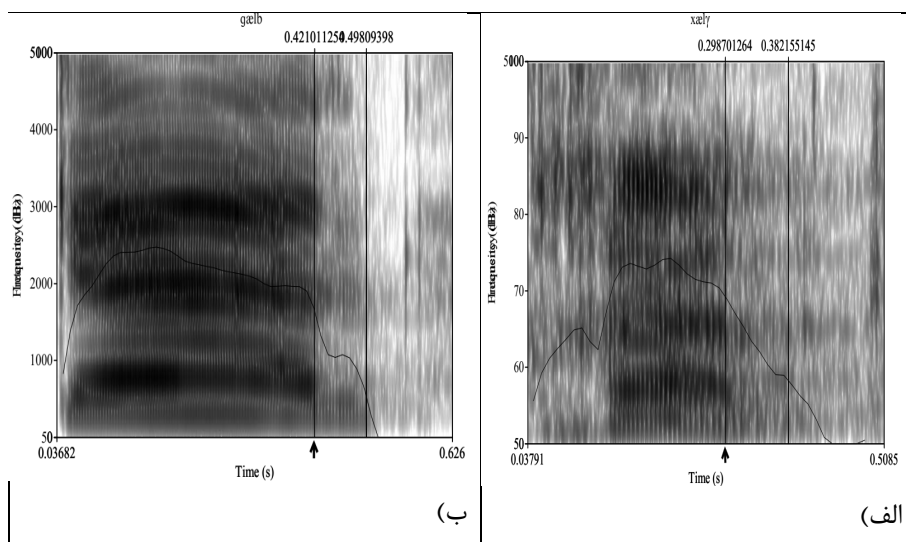
شکل (۱۷) طیف‌نگاشت الف) مربوط به زنجیره آوایی /xæly/ تولیدشده توسط یکی از گویشوران مرد است. ب) مربوط به زنجیره آوایی /gælb/ تولیدشده توسط یکی از گویشوران زن است.
