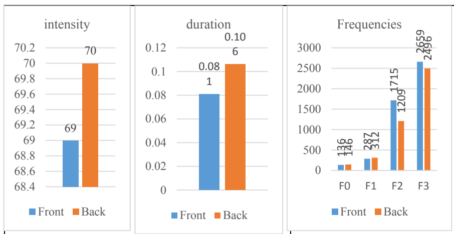
شکل (۴) میانگین فرکانس سازه‌های اول، دوم و سوم [l] بر اساس واکهٔ پس از آن در جایگاه آغاز هجا بعد از همخوان واکدار
